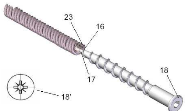
TORNILLO PERFECCIONADO PARA INCRUSTACIÓN DE TUERCAS HELICOIDALES DEFORMABLES
